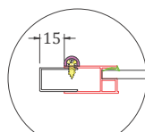
Détail C
