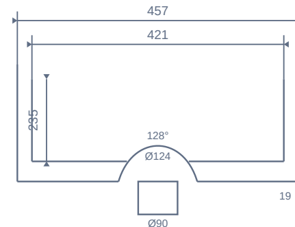
COUPE TRANSVERSALE
