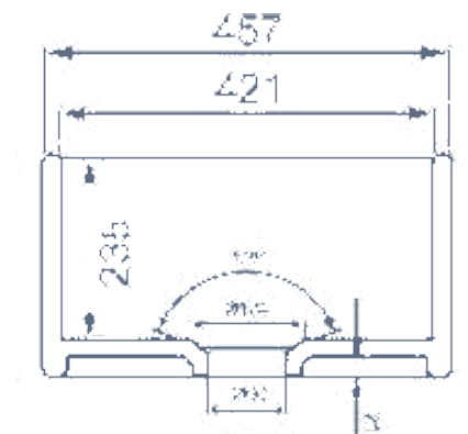
COUPE TRANSVERSALE
