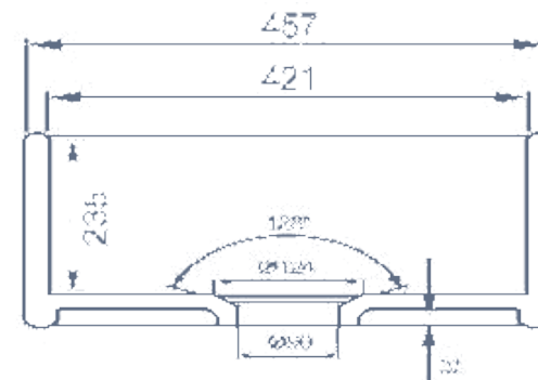
COUPE TRANSVERSALE
