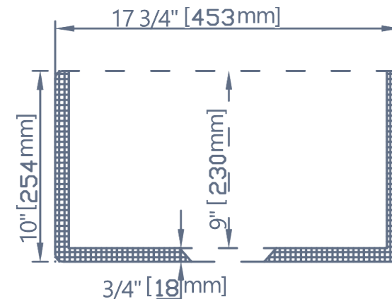
COUPE TRANSVERSALE
